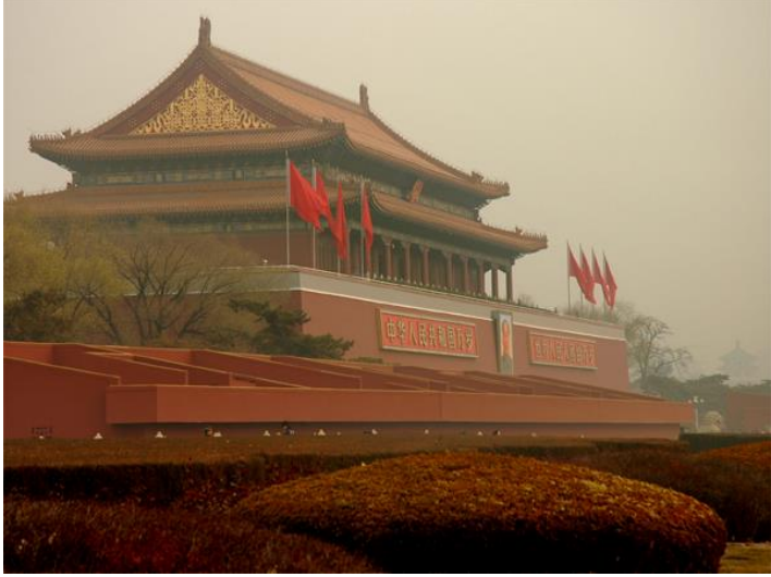
CNN
