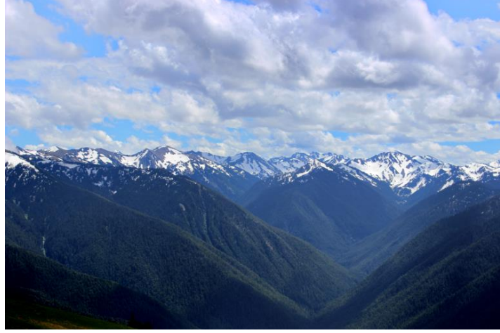
CNN
